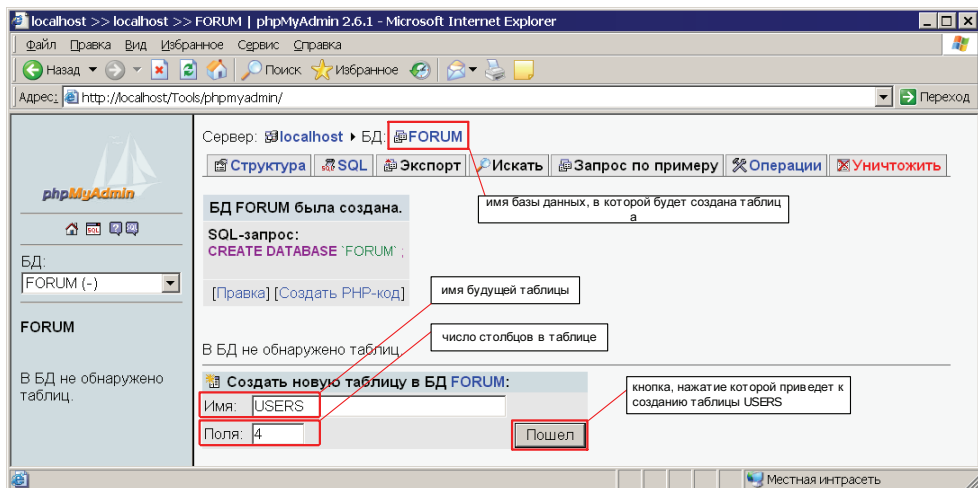
Рис. 10.12. Первый этап создания таблицы: ввод ее имени и числа столбцов, из которых она будет состоять
