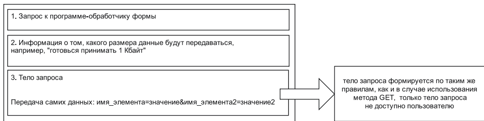
Рис. 7.15. Структура запроса на сервер при передаче формы методом POST
