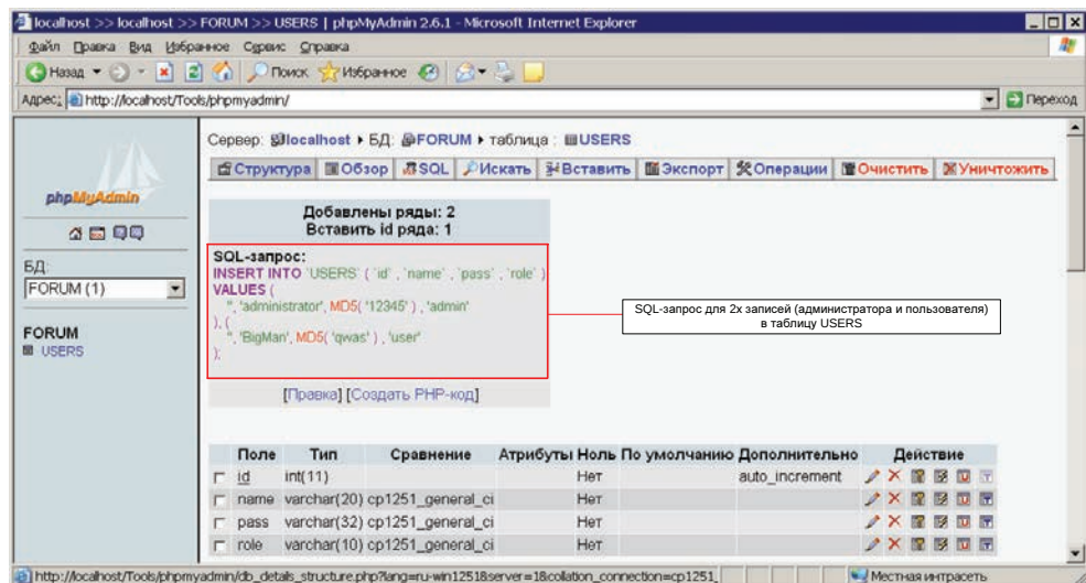
Рис. 10.22. Результат добавления 2 записей в таблицу USERS
