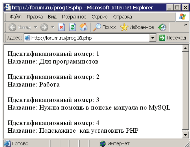
Рис. 10.42. Пример использования функции mysql_fetch_row()
