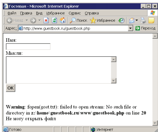
Рис. 9.11. Результат работы гостевой книги в случае отсутствия файла сообщений gost.txt
