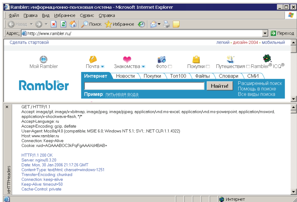
Рис. 8.3. Скрытая информация, которой обмениваются сервер и браузер
