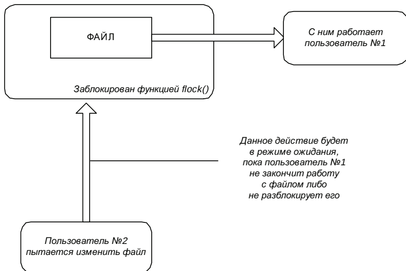
Рис. 6.4. Принцип работы блокировки файла
