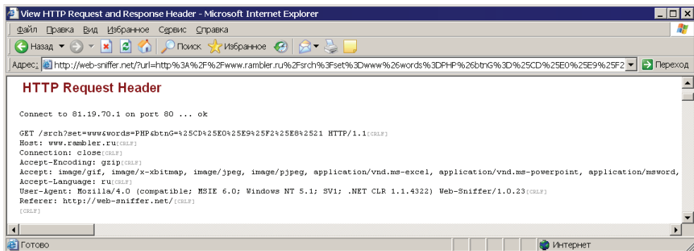
Рис. 8.7. Просмотр отправленных браузером заголовков с помощью сайта www.web-sniffer.net
