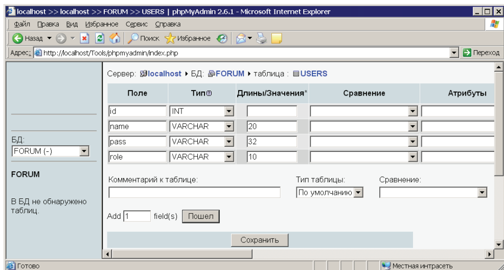
Рис. 10.15. Добавление столбцов в будущую таблицу с именем USERS
