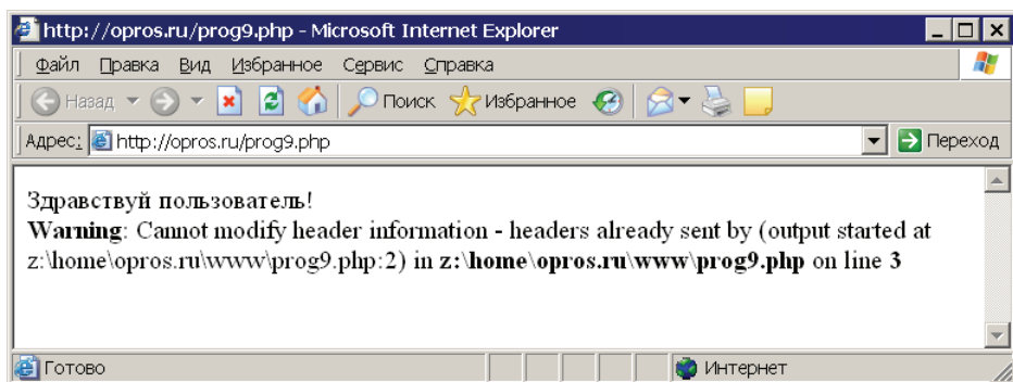
Рис. 9.48. Пример неправильного использования функции setcookie()
