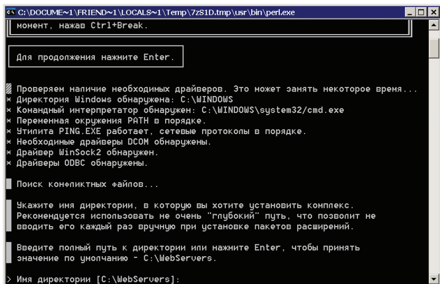
Рис. 4.5. Выбор пути, куда будет установлен Денвер
