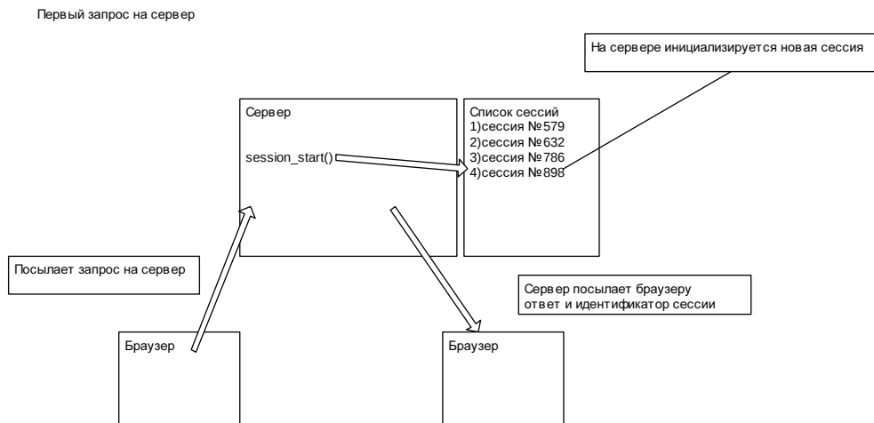
Рис. 9.30. Создание сессии при первом обращении браузера к серверу
