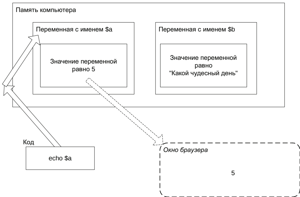
Рис. 5.9. Вывод значения переменной $a с помощью команды echo
