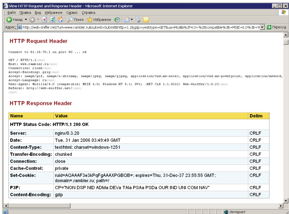
Рис. 8.5. Просмотр скрытой информации с помощью сайта www.web-sniffer.net
