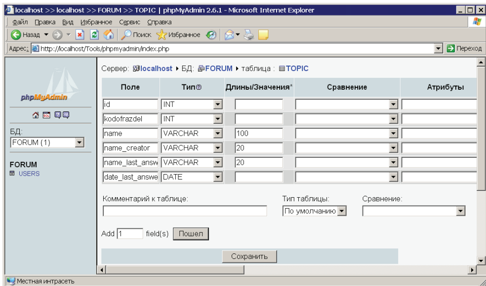
Рис. 10.27. Создание таблицы TOPIC
