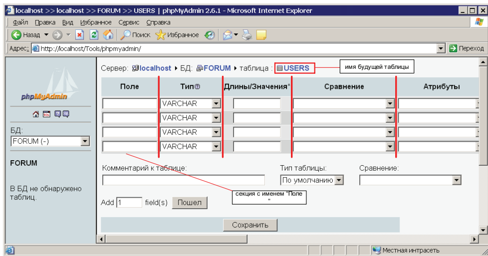
Рис. 10.13. Форма для ввода информации о столбцах для создаваемой таблицы
