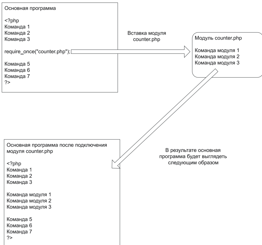
Рис. 6.8. Принцип подключения модуля в программу
