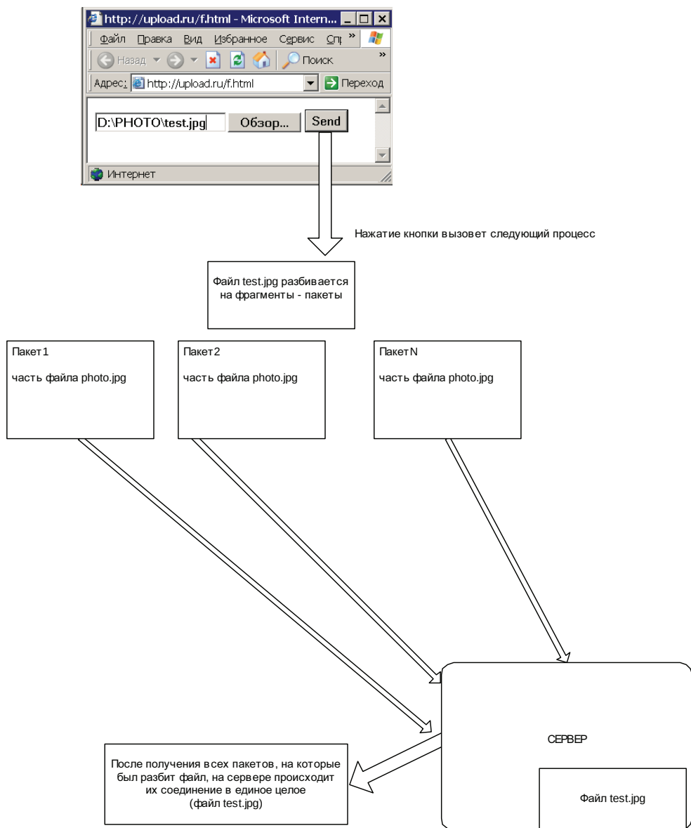
Рис. 9.59. Получение сервером файла, отправленного пользователем через браузер
