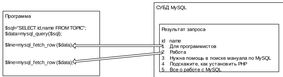
Рис. 10.43. Схема работы функции mysql_fetch_row()
