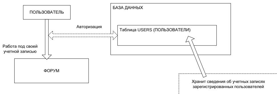
Рис. 10.7. Схема авторизации пользователя на форуме
