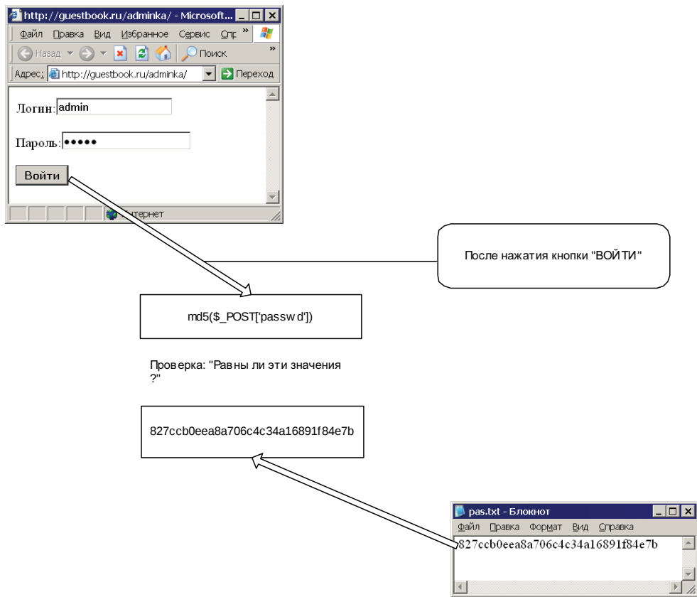
Рис. 9.27. Процесс проверки пароля пользователя, пытающегося зайти в администраторскую часть гостевой книги
