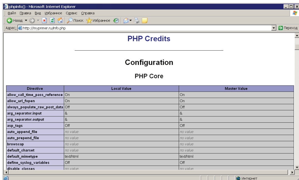
Рис. 4.20. Информация о ядре PHP
