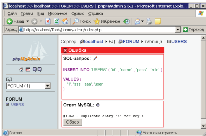
Рис. 10.25. Сообщение об ошибке, возникшее в результате попытки вставить запись с уже существующим значением столбца id
