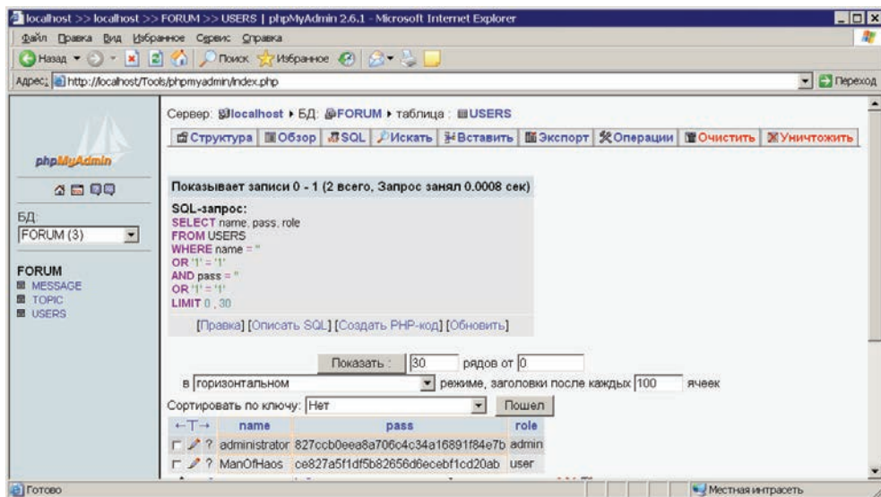
Рис. 10.37. Пример SQL injection
