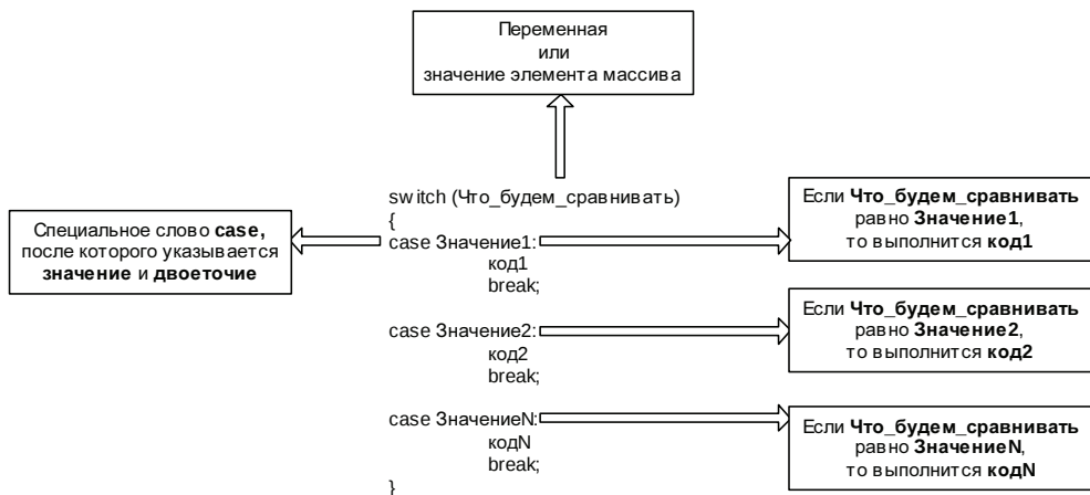
Рис. 9.63. Схема работы конструкции switch
