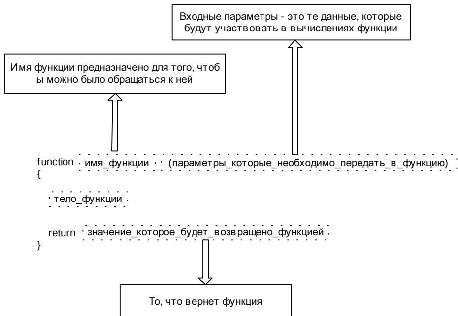
Рис. 9.69. Составные части функции
