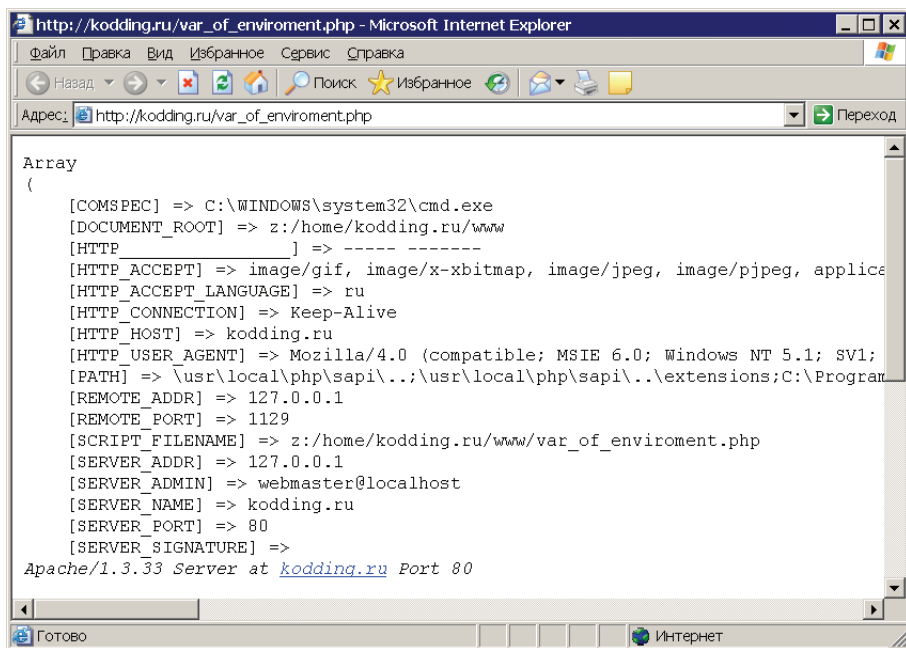
Рис. 5.20. Результат выполнения программы var_of_enviroment.php
