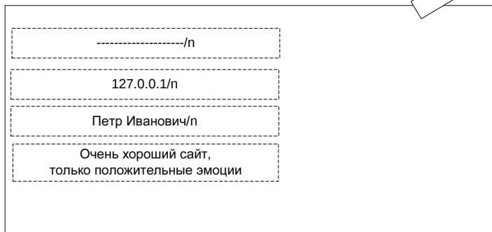
Рис. 9.18. Схема записи в файл gost.txt первого сообщения
